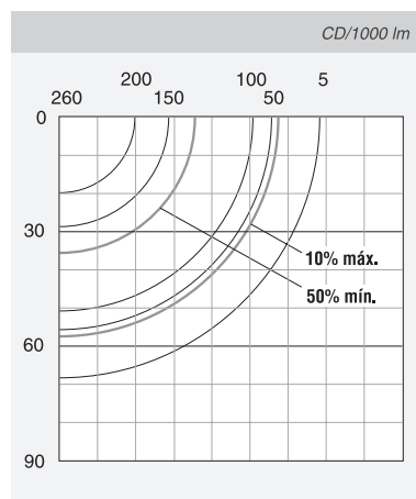
CURVAS ISOCANDELAS
