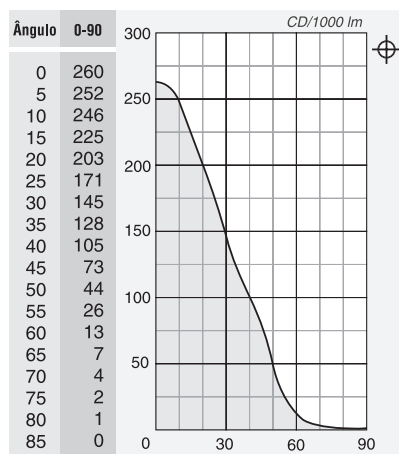
CURVAS CARTESIANAS
